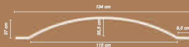
DR-5062 (Ø 120cm)
